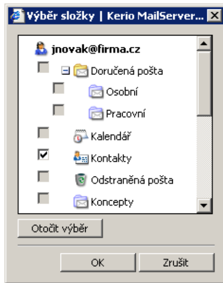
Obrázek 1.89 Výběr složky
