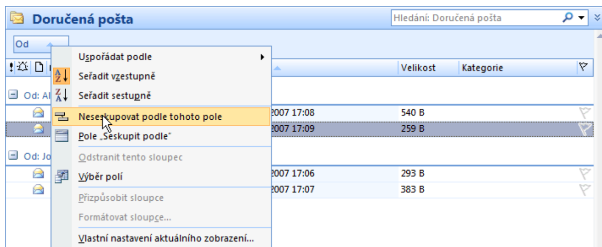
Obrázek 5.27 Odstranění seskupení
