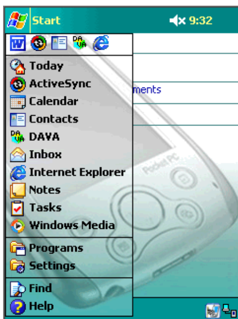
Obrázek 4.1 Nabídka Start
