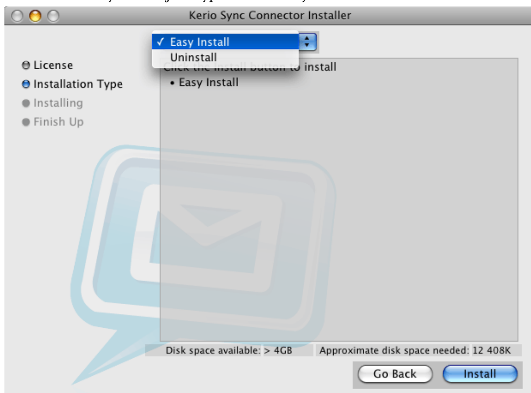
Obrázek 12.2 Nastavení instalace
